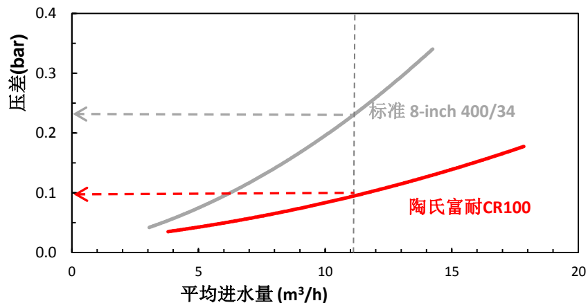
图 1. 陶氏富耐 CR100 与普通反渗透膜相比，膜元件压差随流量的变化趋势
